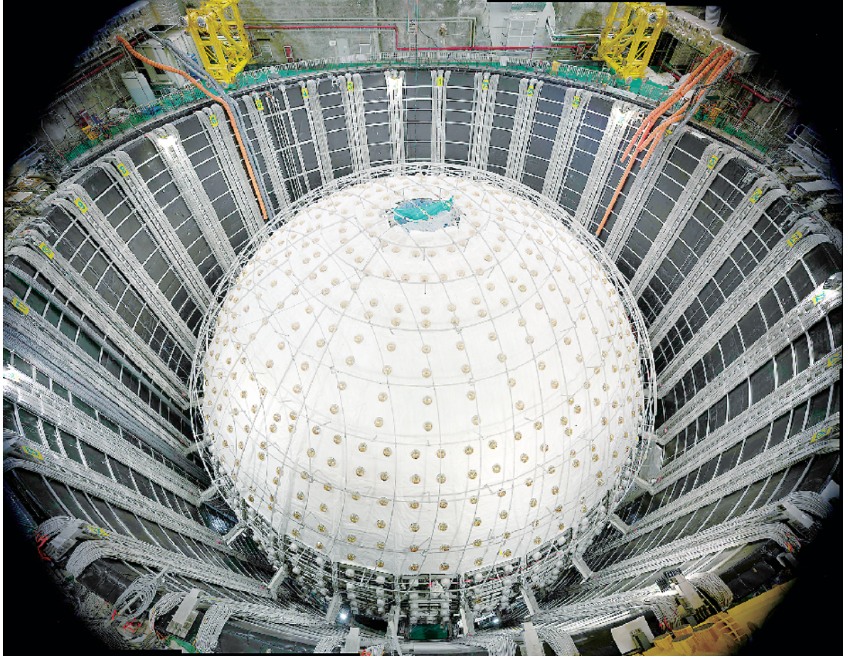
2024年10月9日拍摄的建设中的江门中微子实验中心探测器(拼接照片)。
